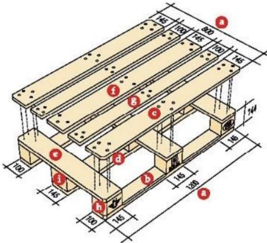
Godkända mått i mm
